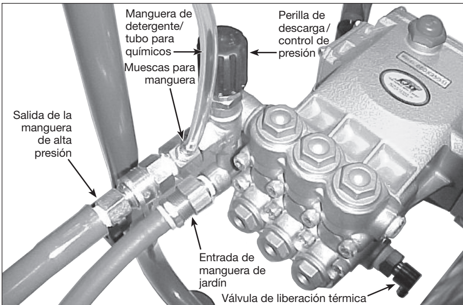
Figura 12 - Conexión de la bomba (Se muestra PW4070 - los demás modelos son similares)
